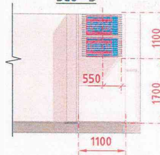
Вид Б
