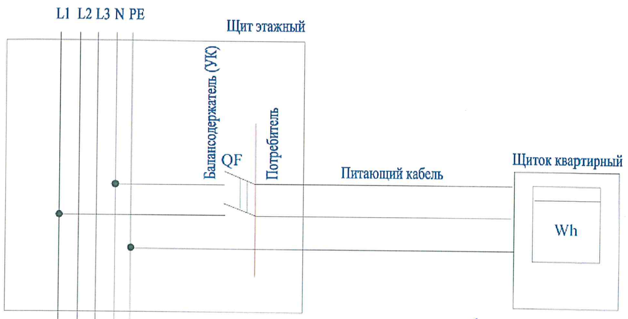
Граница балансовой принадлежности и эксплуатационной ответственности сторон
