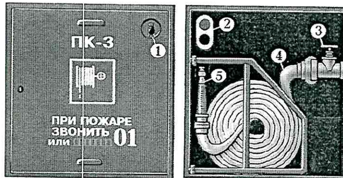
Рис. 10. Внутренний пожарный кран: 1 — место хранения ключа; 2 — пульт дистанционного включения насосовысителя; 3 — пожарный кран; 4 — пожарный рукав; 5 — ствол
