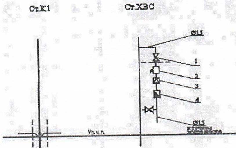
Рисунок № 1. Схема разграничения ответственности по ХВС и канализации.
